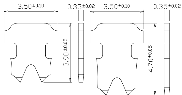
“ 2 ” : 2 PRONGS FOR STRANDED WIRE 多芯線用二叉型金片
