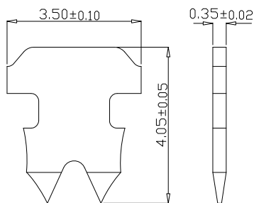
“S” : 2 PRONGS FOR STRANDED WIRE 多芯線用二叉型金片
